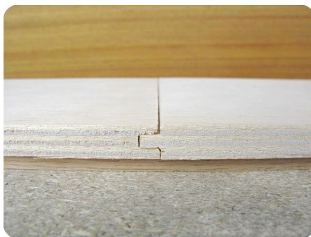
sistema di supporto brevettato a mattonella: particolare dell'incastro degli elementi di supporto in fase di incollaggio alla lamella
